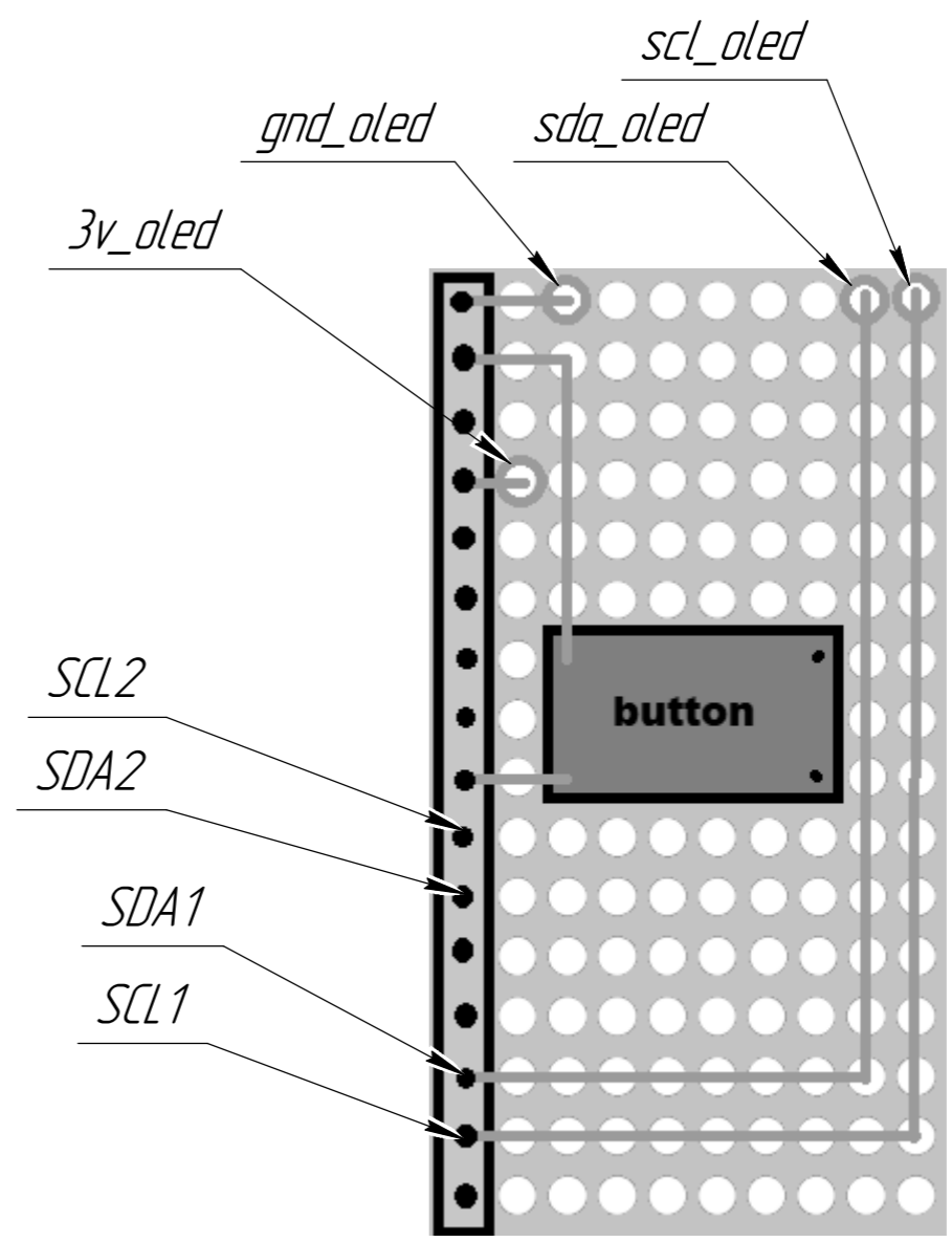
Модуль с кнопкой и распиновкой для oled
